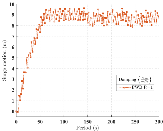
شکل ۲۱- حرکت سرج موج شکن در پریود ۵ ثانیه با مبدل ۱ متر و چیدمان ۱
