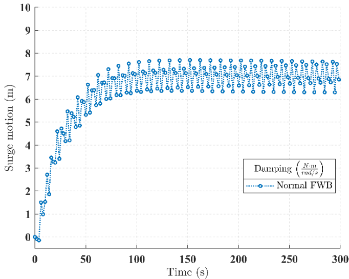
شکل ۲۰- حرکت سرج موج شکن در پریود ۵ ثانیه بدون مبدل
